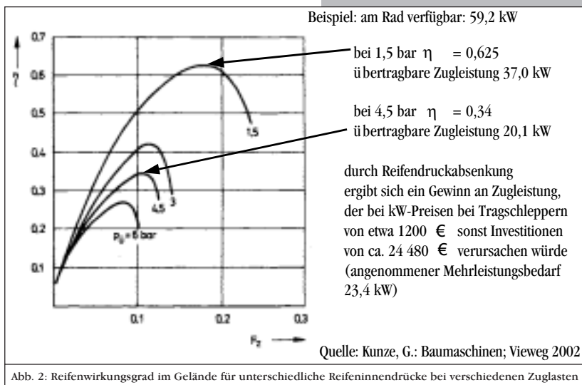
Abb. 2: Reifenwirkungsgrad im Gelände für unterschiedliche Reifeninnendrucke bei verschiedenen Zuglasten
