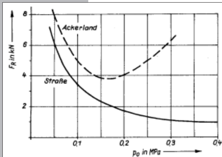
Abb.1: Rollwiderstand von Reifen in Abhängigkeit vom Innendruck auf der Straße und im Gelände
