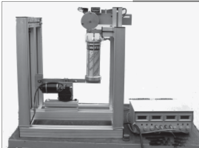
Abb. 3: Prüfstand zur Bestimmung der Ergiebigkeit von Sprühdosen
