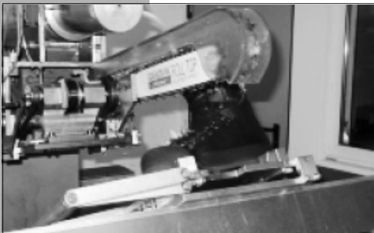
Beispiel: Prüfung von Schnittschutz in Sicherheitsschuhen
